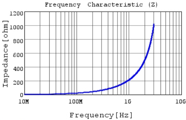
LQW15AN33NG0Z |Z|
