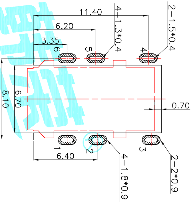
P.C.B LAYOUT
