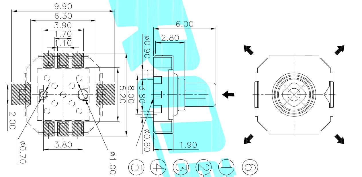
PCB Layout(Pattern Side)
