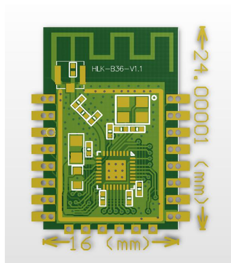
图 1 HLK-B36 封装大小
