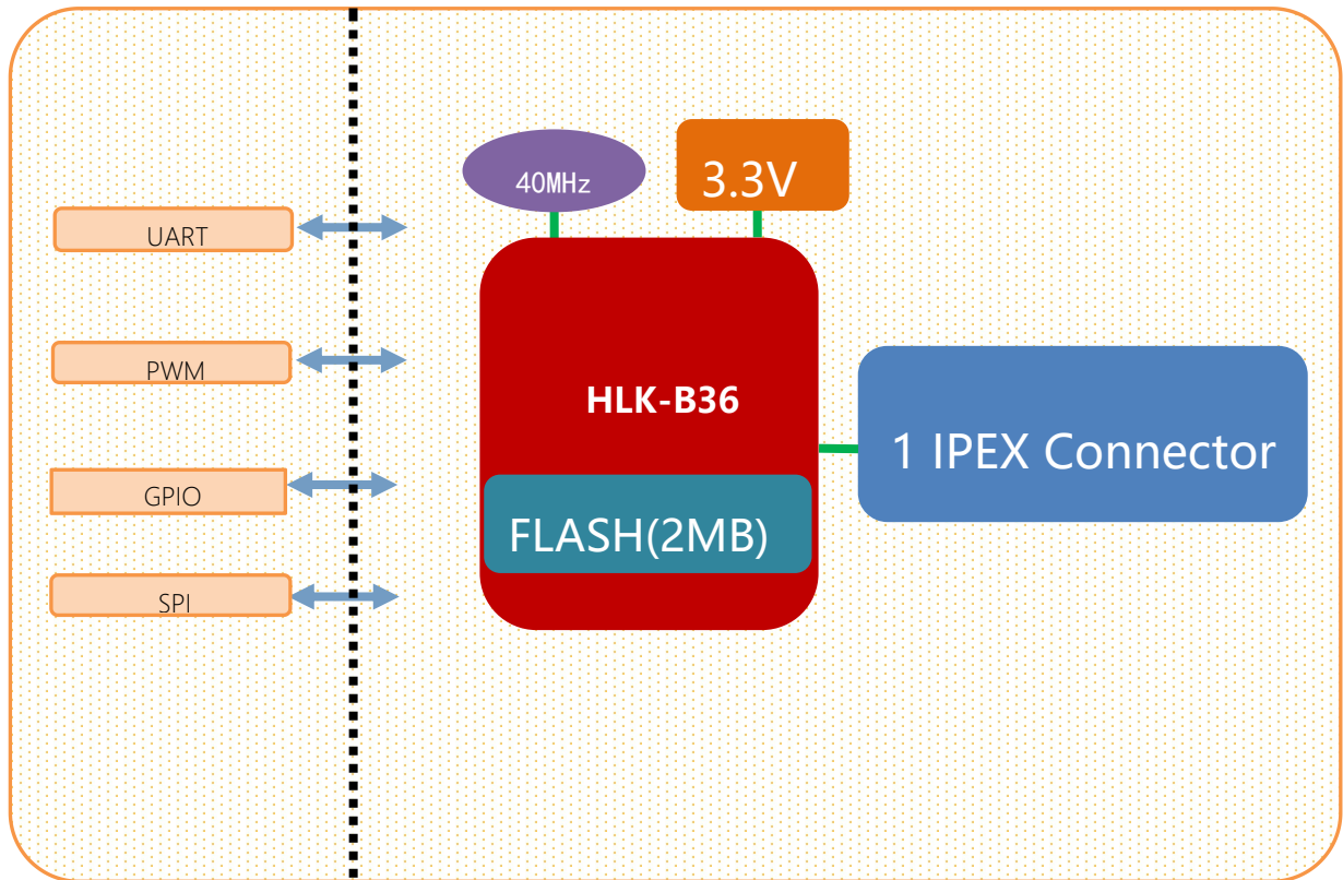
图 2. HLK-B36 模块架构图
