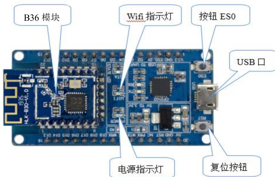
图 3 底板说明图
