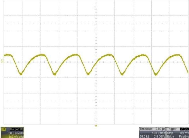
Noise V_{IN}=40V , I_o=2A , 5~20MHz Bandwidth
