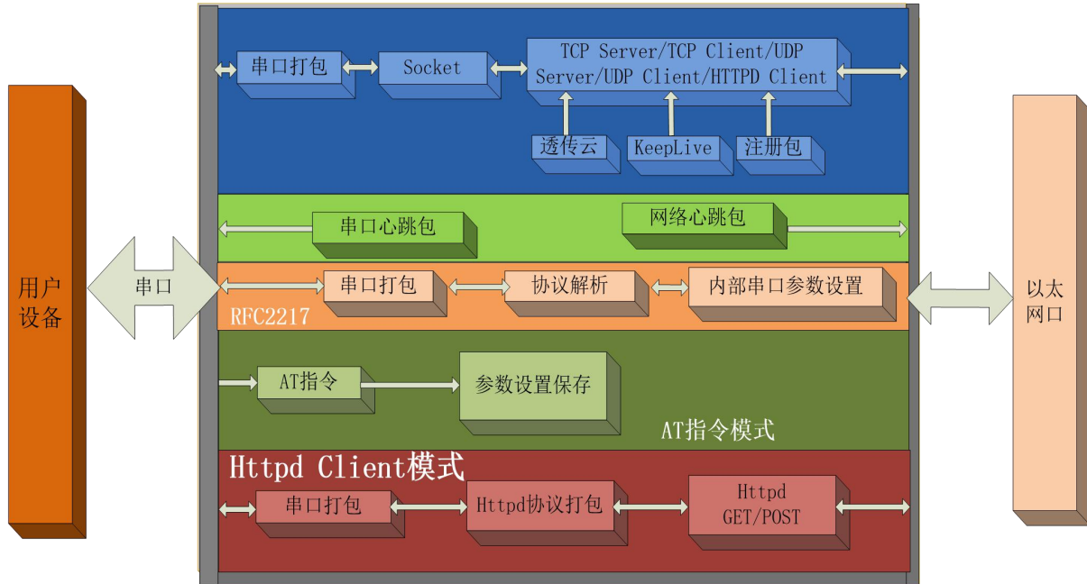
图 7. 301 功能框图
