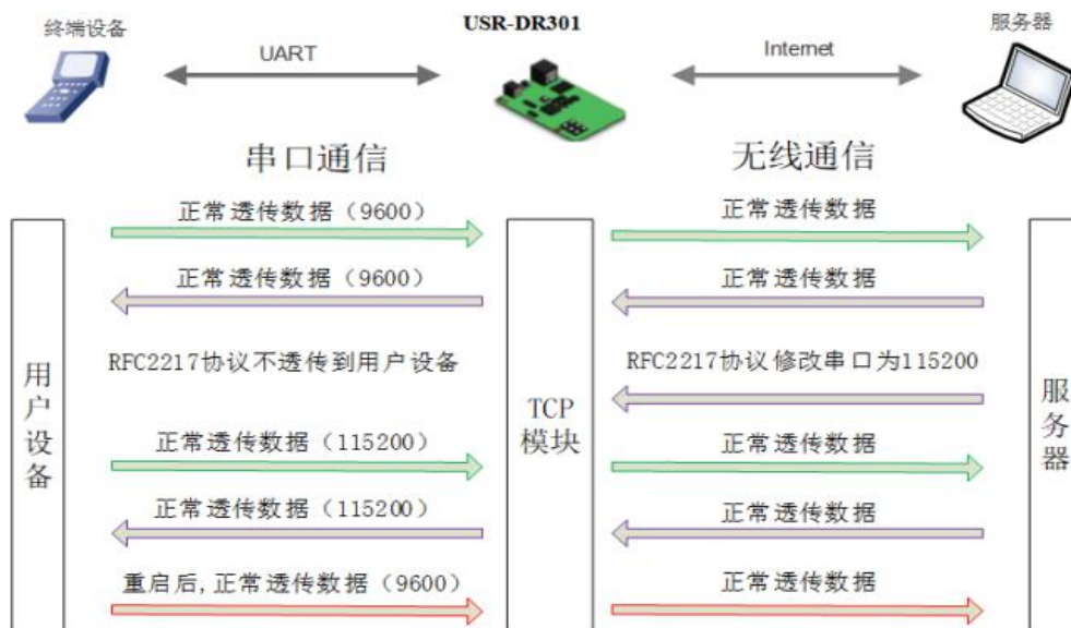
图 21. 类 RFC2217 功能框图
