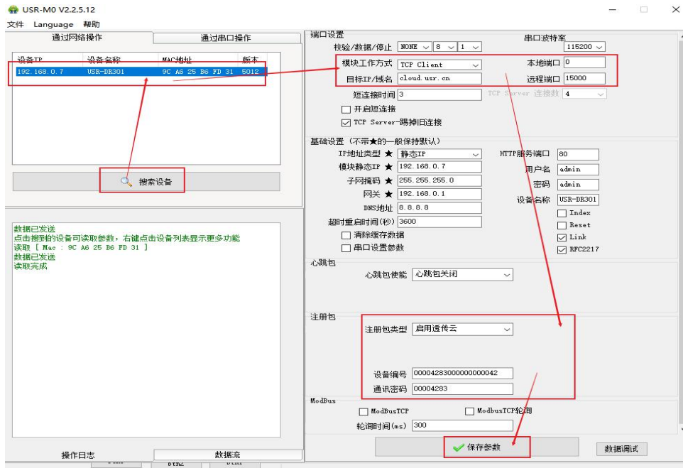
图 29. 透传云设置图示
