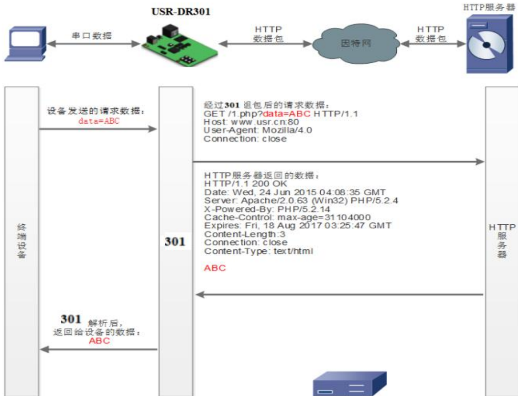
图 16. Httpd Client 模式说明
