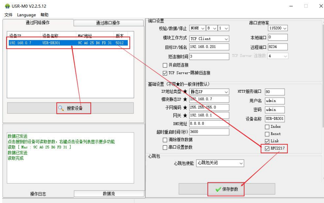
图 20. 类 RFC2217 功能设置
