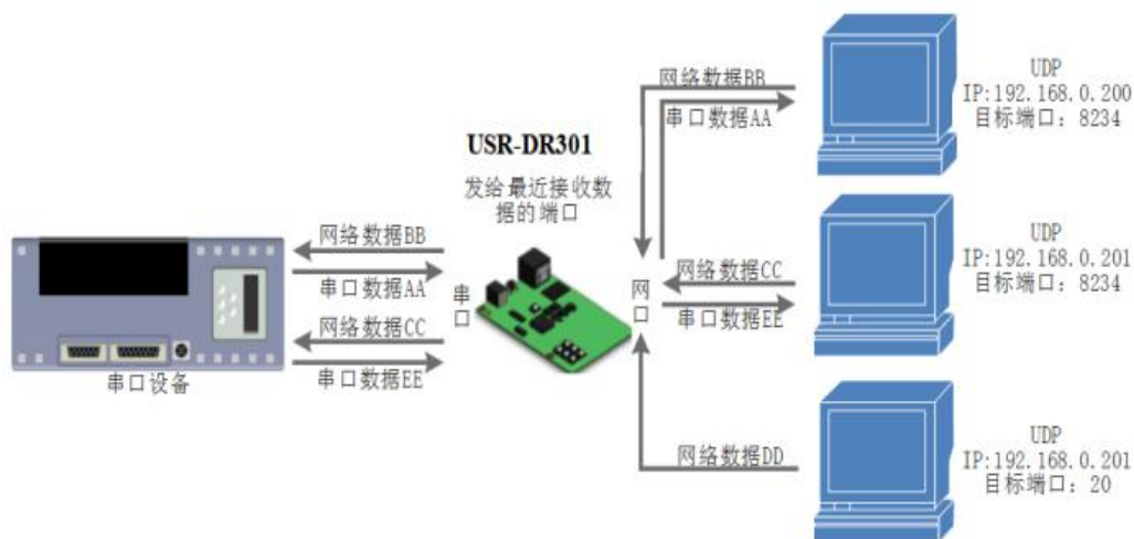
图 15. UDP Server 模式
