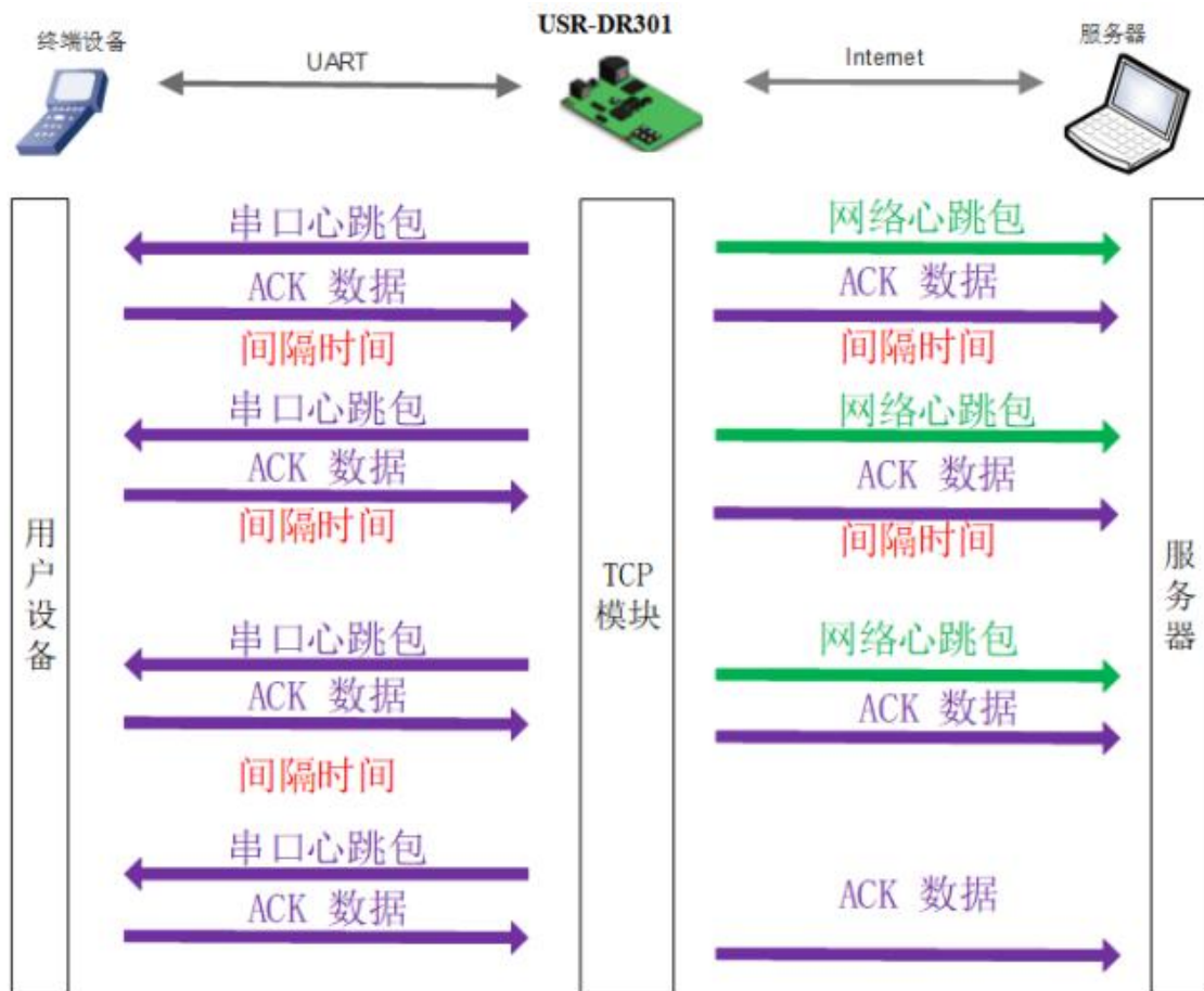
图 23. 心跳包功能示意图
