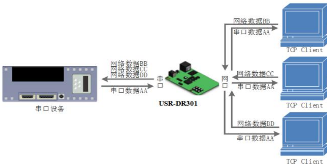
图 13. TCP Server 模式说明
