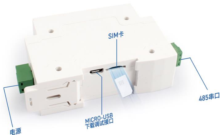
图1. 接口说明
