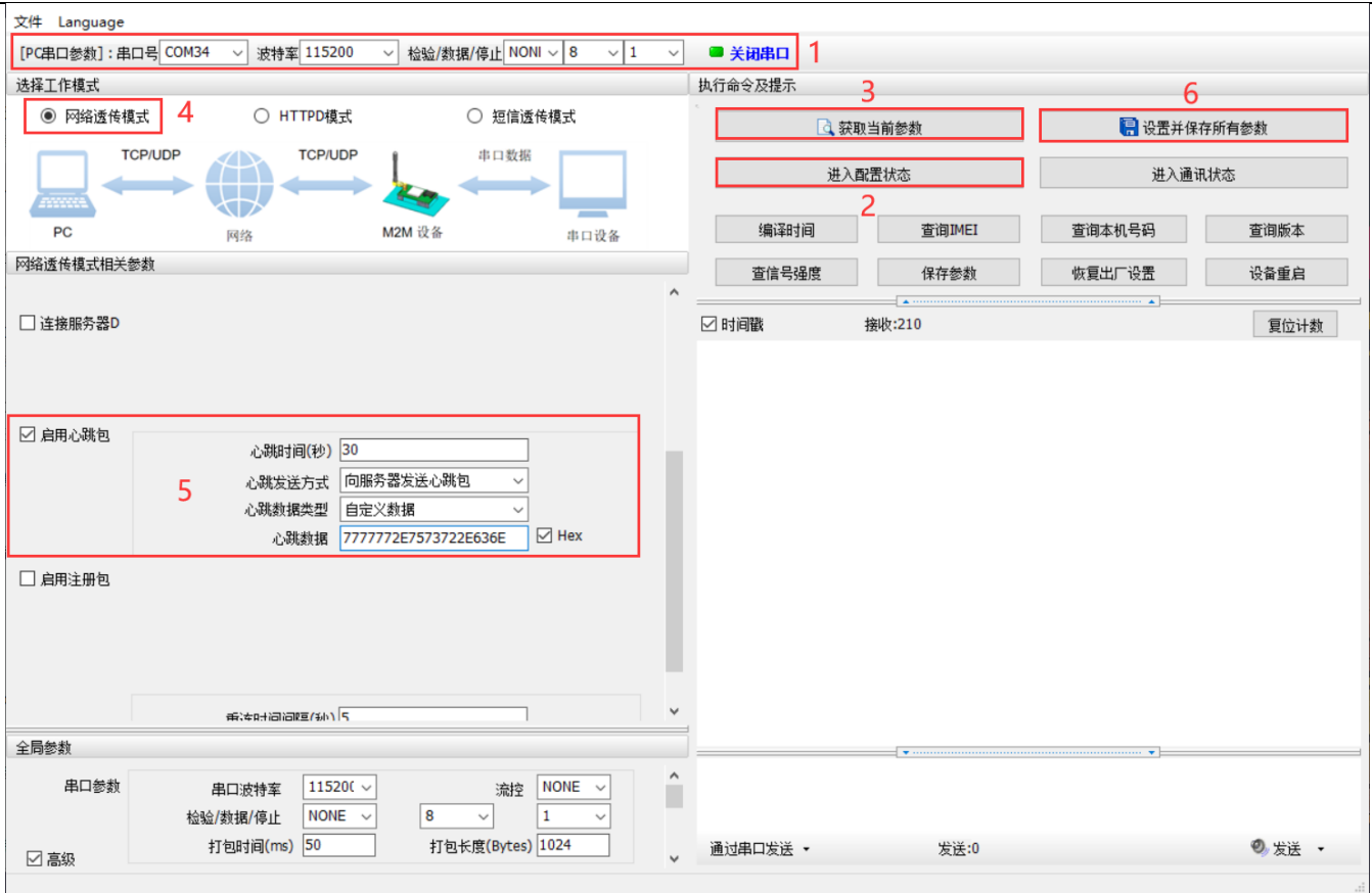
图11. 设置软件示意图
