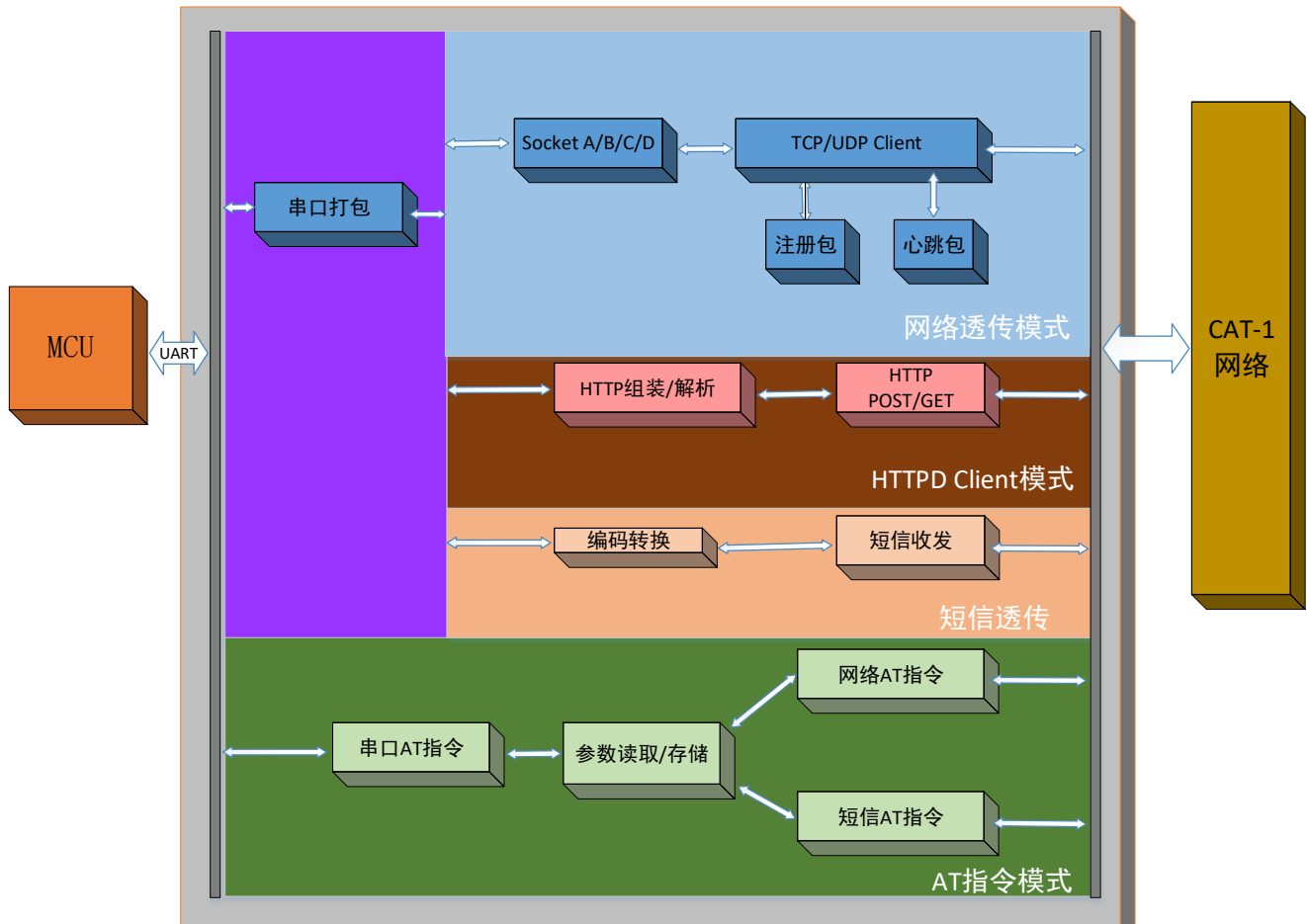
图3. 功能框图
