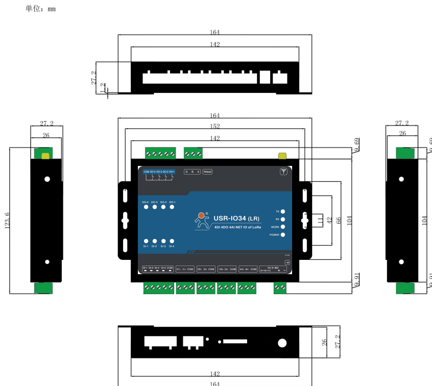
图 11 USR-IO34-LR 尺寸图
