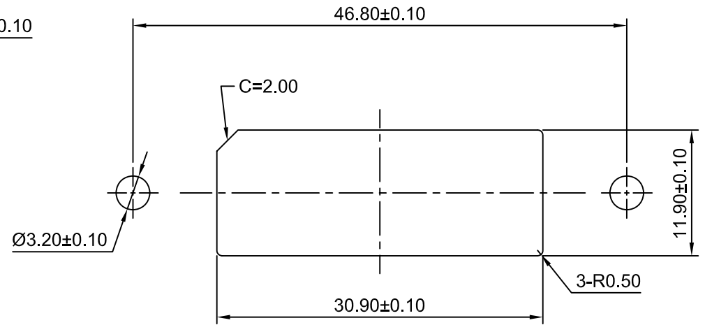
P.C.B LAYOUT
