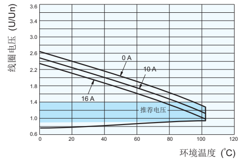
线圈工作范围曲线 (DC)
