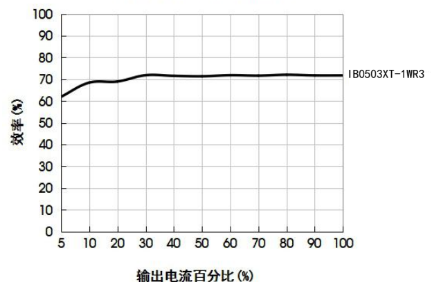
效率Vs输出负载 ( V_{in}=5\text{V} )
