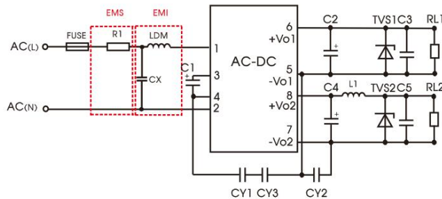
推荐电路 2
