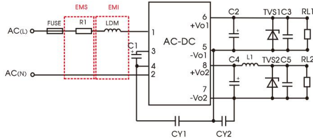
推荐电路 1
