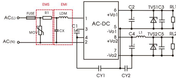
推荐电路 3
