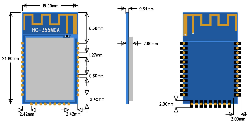
图 2 模块尺寸图
