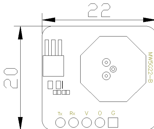
图 4.2 MW5G22-B 模块尺寸图
