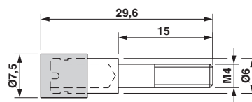
尺寸图
