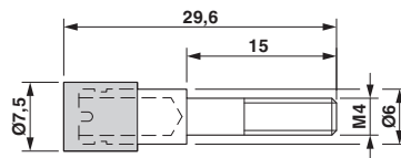
尺寸图
