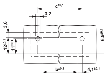
钻孔图
