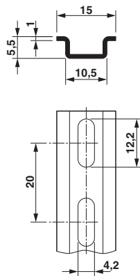
尺寸图
