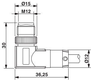
尺寸图
