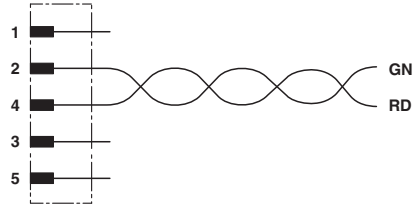
电路图
