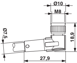
尺寸图
