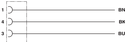
M8针式/孔式触点分配
