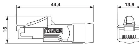
尺寸图
