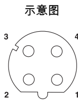
M12孔式连接器引脚分配，4芯，D编码，插座侧
