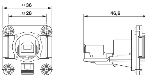
尺寸图
