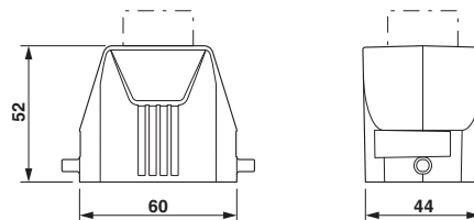
尺寸图
