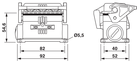
尺寸图
