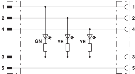
带有3个LED的M12针式/孔式连接器的触点分配
