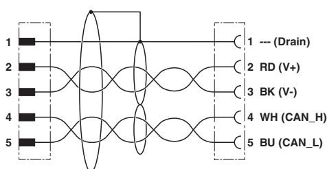
电路图
