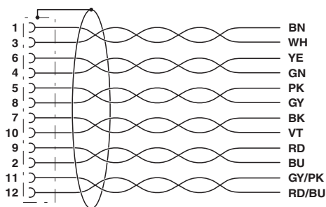
电路图
