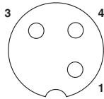
M12孔式连接器引分配，3芯，A编码，插座侧视图
