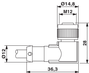
尺寸图
