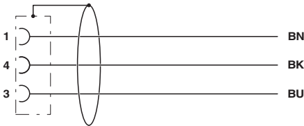
电路图
