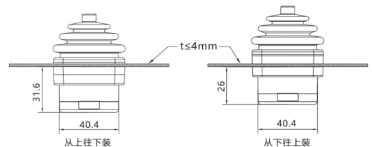
机械安装图
